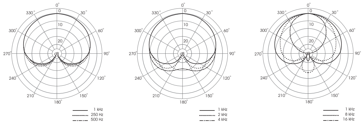
Polardiagramme
